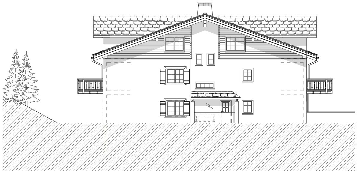
Nord - Fassade
