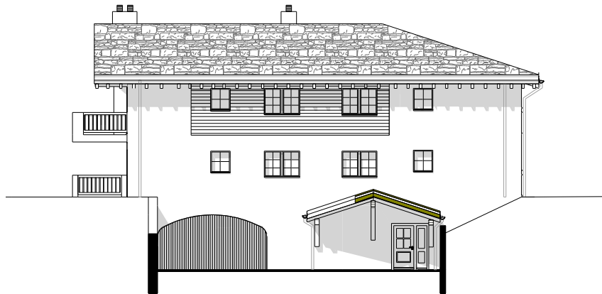
Ostfassade
