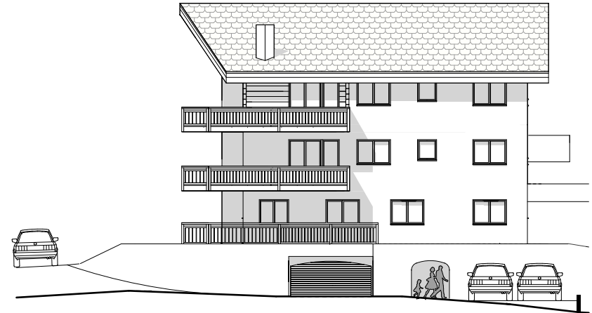
Ost - Fassade
