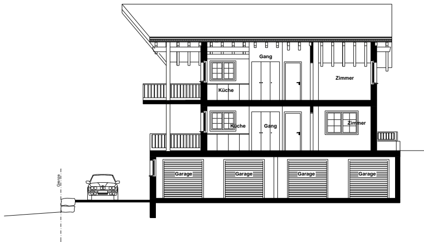
Haus A Längsschnitt
