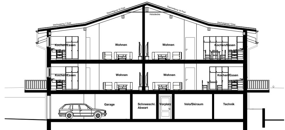
Haus A Querschnitt
